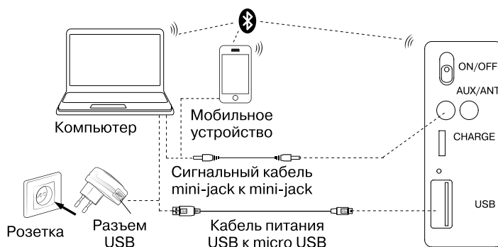
Рис. 2. Схема подключения
